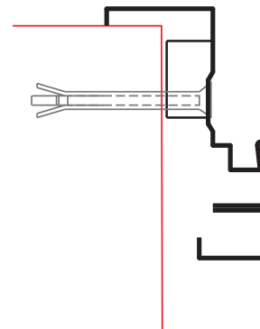
Karmtype hjørne
