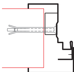
Karmtype vægomslyttende
